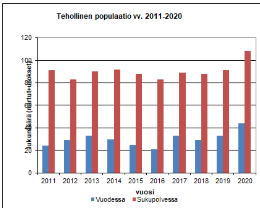
Kuva 3. Gööttien tehollinen populaatiokoko vuodessa ja sukupolvessa kymmenen vuoden tarkastelujakson aikana.
