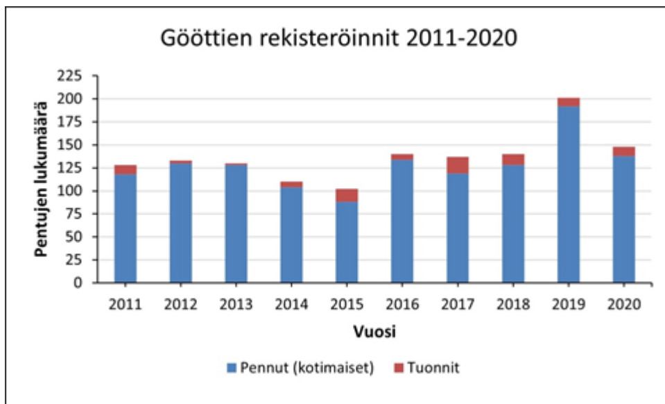
Kuva 1. Gööttien rekisteröintimäärät/vuosi kymmenen vuoden tarkastelujaksolla.
